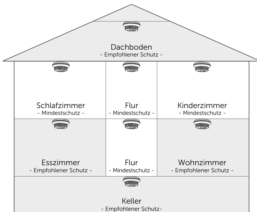
Abbildung 38: Installationshinweise Homematic IP Rauchwarnmelder mit Q-Label
